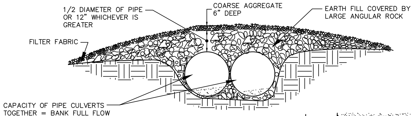
ELEVATION
